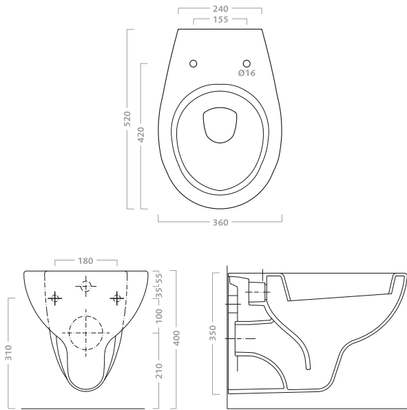
vaso sospeso vaso a cacciata con scarico a parete (p). funziona con 6 litri. peso kg ca. 14,5 codice descrizione 63312 vaso sospeso 63760 sedile in termoindurente 20969 supporto per muro non portante 20961 supporto per muro portante
