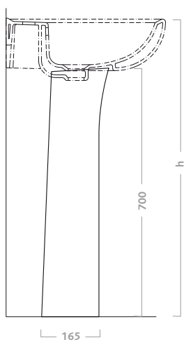
colonna da abbinare a lavabo 55 cod. 63050 h840, 60 cod. 63040 h845, 65 cod. 63030 h855. peso kg ca. 8,5 codice descrizione 63150 colonna
