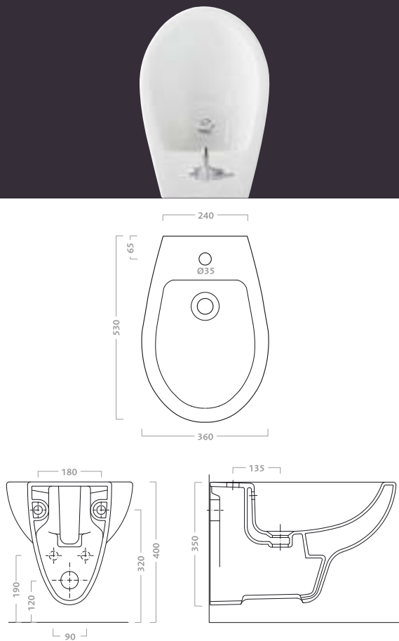
bidet sospeso disponibile per rubinetteria monoforo. peso kg ca. 14 codice descrizione 63255 bidet sospeso 20968 supporto per muro non portante 20961 supporto per muro portante
