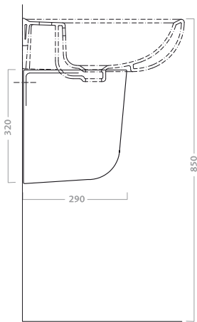
semicolonna da abbinare a lavabo 55 cod. 63050, 60 cod. 63040, 65 cod. 63030. peso kg ca. 5 codice descrizione 63160 semicolonna
